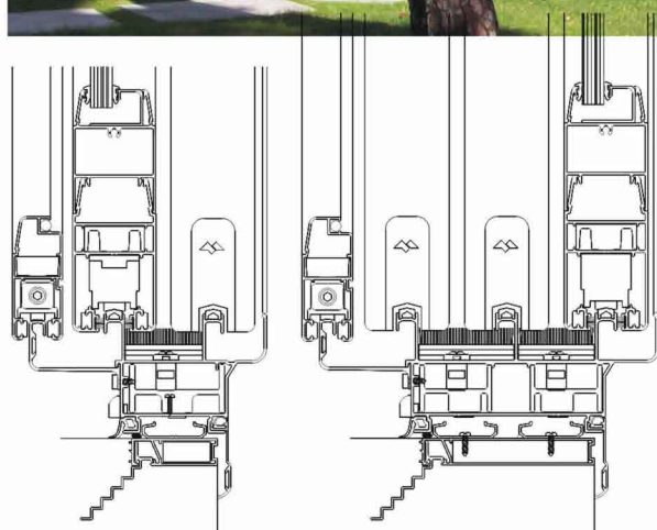
detalle corrediza 2 guias-vertical
