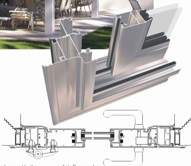
detalle corrediza 3 guias-vertical
